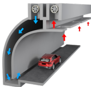
VENTILAÇÃO TRANSVERSAL
