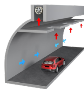
VENTILAÇÃO SEMITRANSVERSAL
