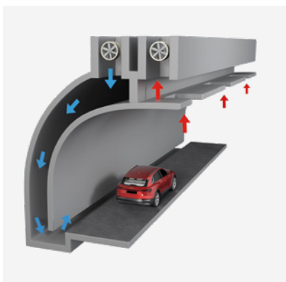
VENTILAÇÃO TRANSVERSAL
