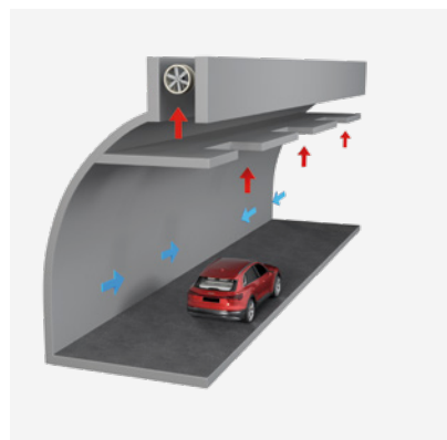
VENTILAÇÃO SEMITRANSVERSAL
