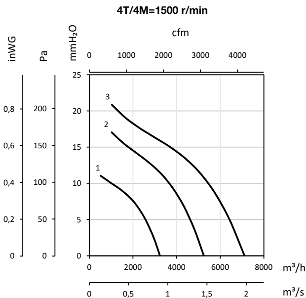
1 : HCH-35-4T 2 : HCH-40-4T-0.33
