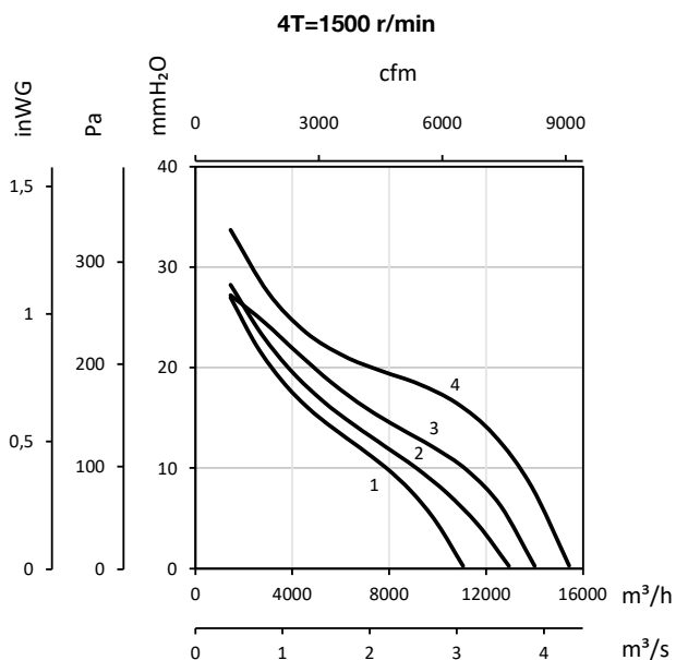
1 : HCH-56-4T-0.75 2 : HCH-56-4T-1
