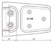
Dobradiça N 149
